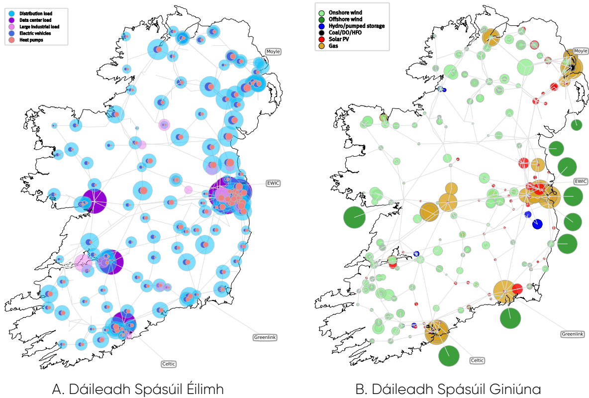
Fíor 12: Réamh-mheastacháin éilimh agus soláthair amach anseo go dtí 2030
