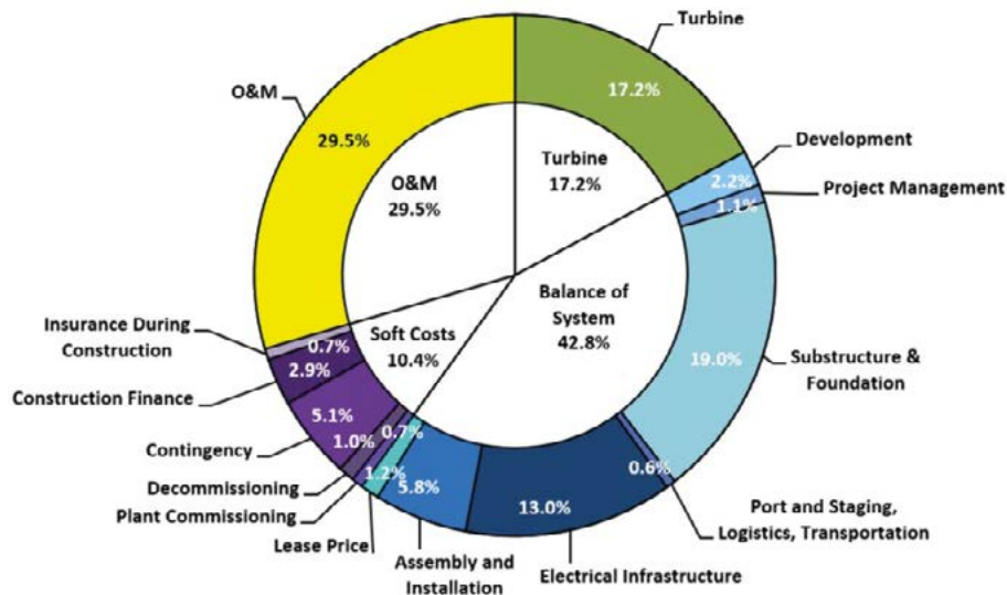
Fíor 11: Ranniocáíocht MITF (meánchostas iomlán táirgthe fuinnimh) Leibhéal Comhpháirte do thionscadal tagartha eischósta ar snámh ag feidhmiú ar feadh 25 bliana (Foinse: An tSaotharlann Náisiúnta um Fhuinneamh In-athnuaite 42 )
