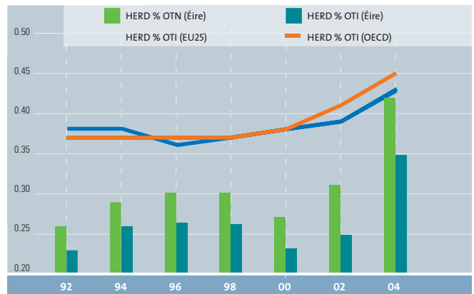
Figiúr 10 Higher Education Expenditure on R&D (% gníomhaíocht gheilleagrach) 1992-2004 (e)
