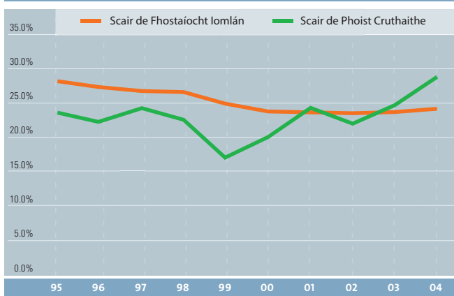
Figiúr 4 Scair de Fhostaíocht i gComhlachtaí Tacaíthe ag Gníomhaireacht Réigiún an TLI freagrach as seo
