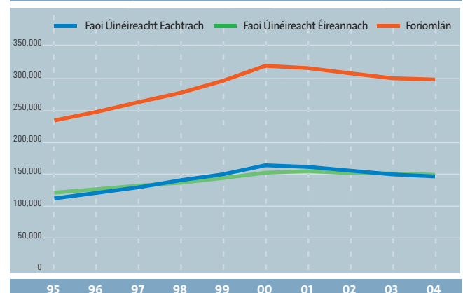
Figiúr 2 Fostaíocht Bhuan Lánaimseartha 1995-2004 Déantúsaíocht agus Seirbhísí Trádáilte go hidirnáisiúnta/Seirbhísí Airgeadais
