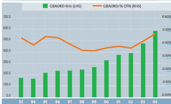
Figiúr 11 Deontais Rialtais Dáilte do Thaighde agus Fhorbairt (1993-2004)
