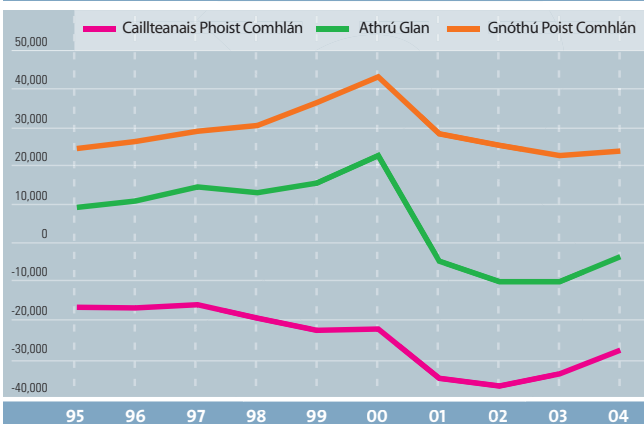
Figiúr 3 Poist a Ghnóthú, a Chailliúint agus Athrú Glan i bhFostaíocht Bhuan Lánaimseartha 1995-2004 Déantúsaíocht agus Seirbhísí Trádáilte go hidirnáisiúnta/Seirbhísí Airgeadais
